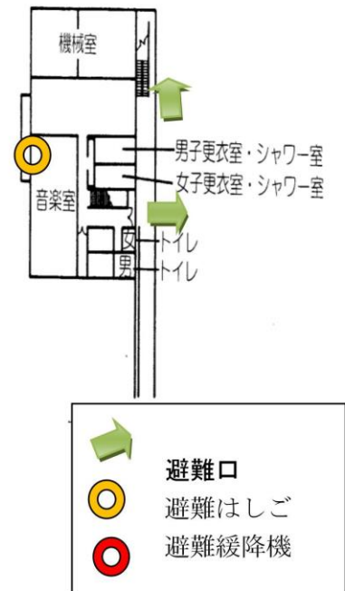
3 階平面
